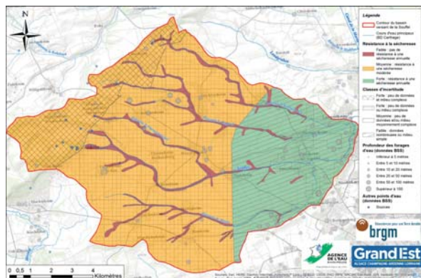
Cartographie de la résistance à la sécheresse des entités hydrogéologique du bassin versant de la Souffel. ©BRGM
